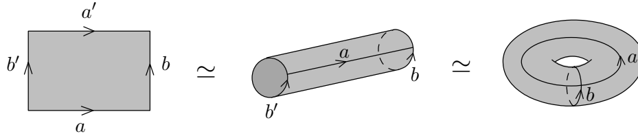
Fig. 1.12. Gluing a torus
