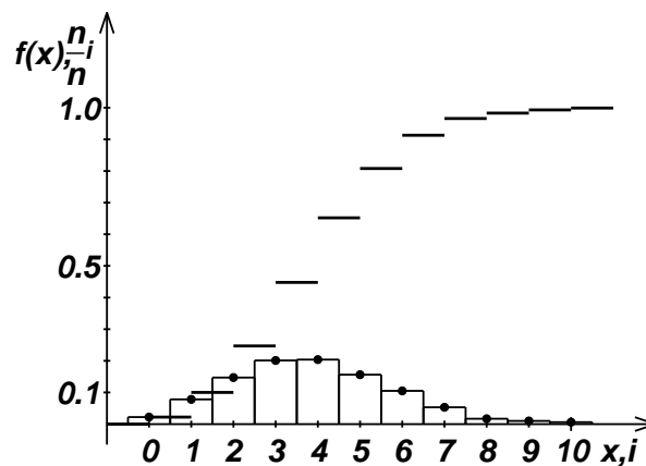
Abbildung 1: Empirische Wahrscheinlichkeitsverteilungsfunktion f(x) nach (14.1) und Histogramm
